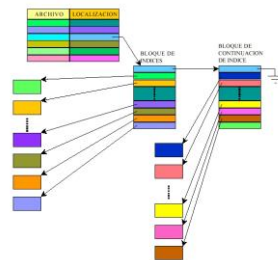
Figura 1.5: Funcionamiento de bloques de índices.
